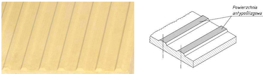
Rys. 1a. Płytki kierunkowe symetryczne - prowadząca - szczegóły powierzchni
