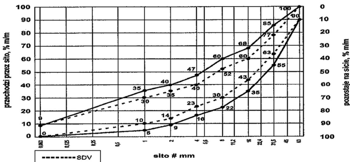
Rys. 3. Krzywe graniczne uziarnienia mieszanki kruszywa niezwiązanego 0/63 mm do warstw
