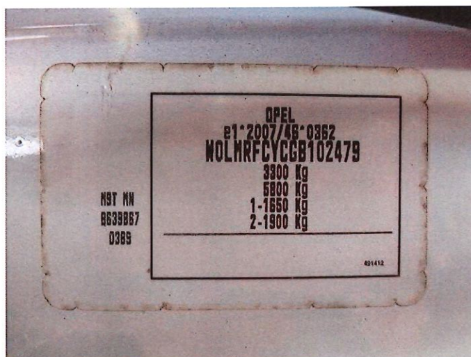
Tabliczka znamionowa.
