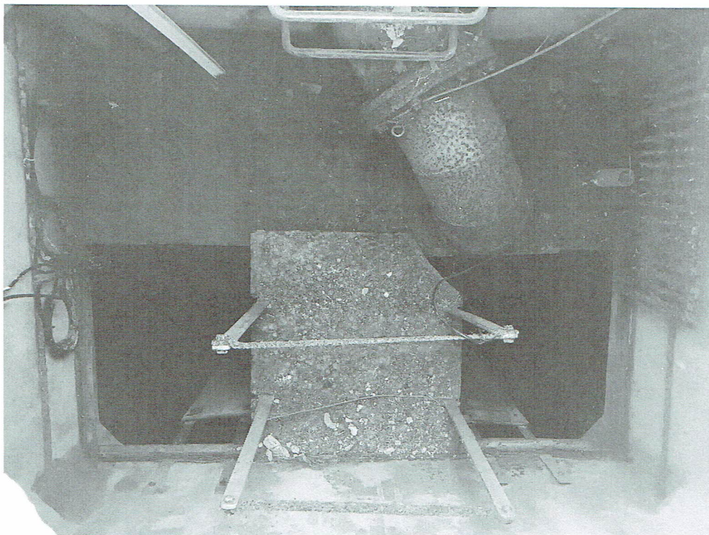
Fot.3 Zejście do zbiornika: komora przejściowa – widok na podest (spoczywający na przegrodzie wewnętrznej zbiornika) oraz widok na otwory obydwu komór zbiornika
