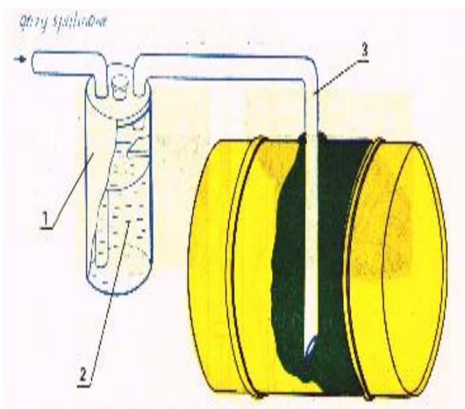
Cięte lub spawane pojemniki mogące zawierać gazy lub pary palnych cieczy należy przed przystąpieniem do prac wypełnić gazem obojętnym np. gazami spalinowymi poprzez urządzenie do wylapywania iskier: 1- urządzenie do wylapywania iskier, 2- woda, 3- przewód
