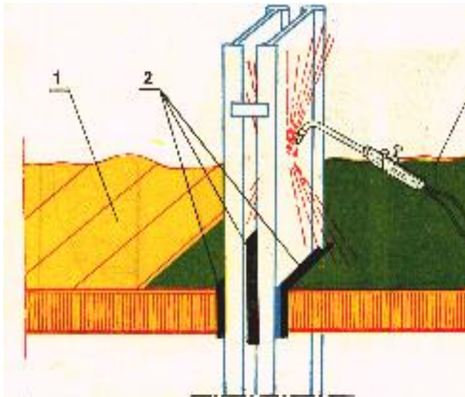
Sposób prawidłowego zabezpieczenia spawania metalowego elementu konstrukcji, przechodzącego przez drewniany strop: 1- drewniany strop, 2- niepalne uszczelnienie, 3- koc gaśniczy
