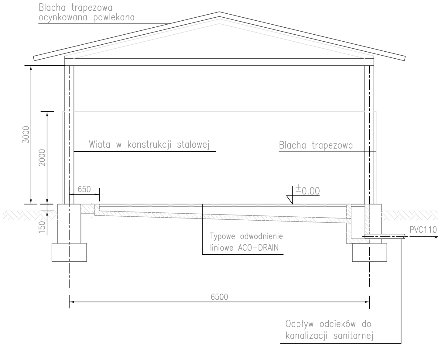
PRZEKRÓJ B-B
