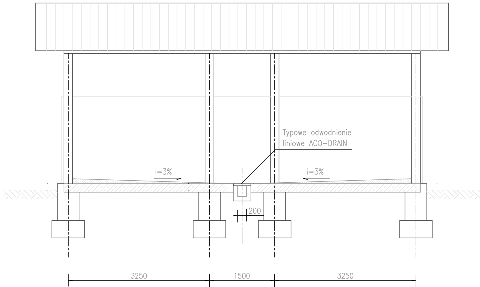
PRZEKRÓJ A-A.
