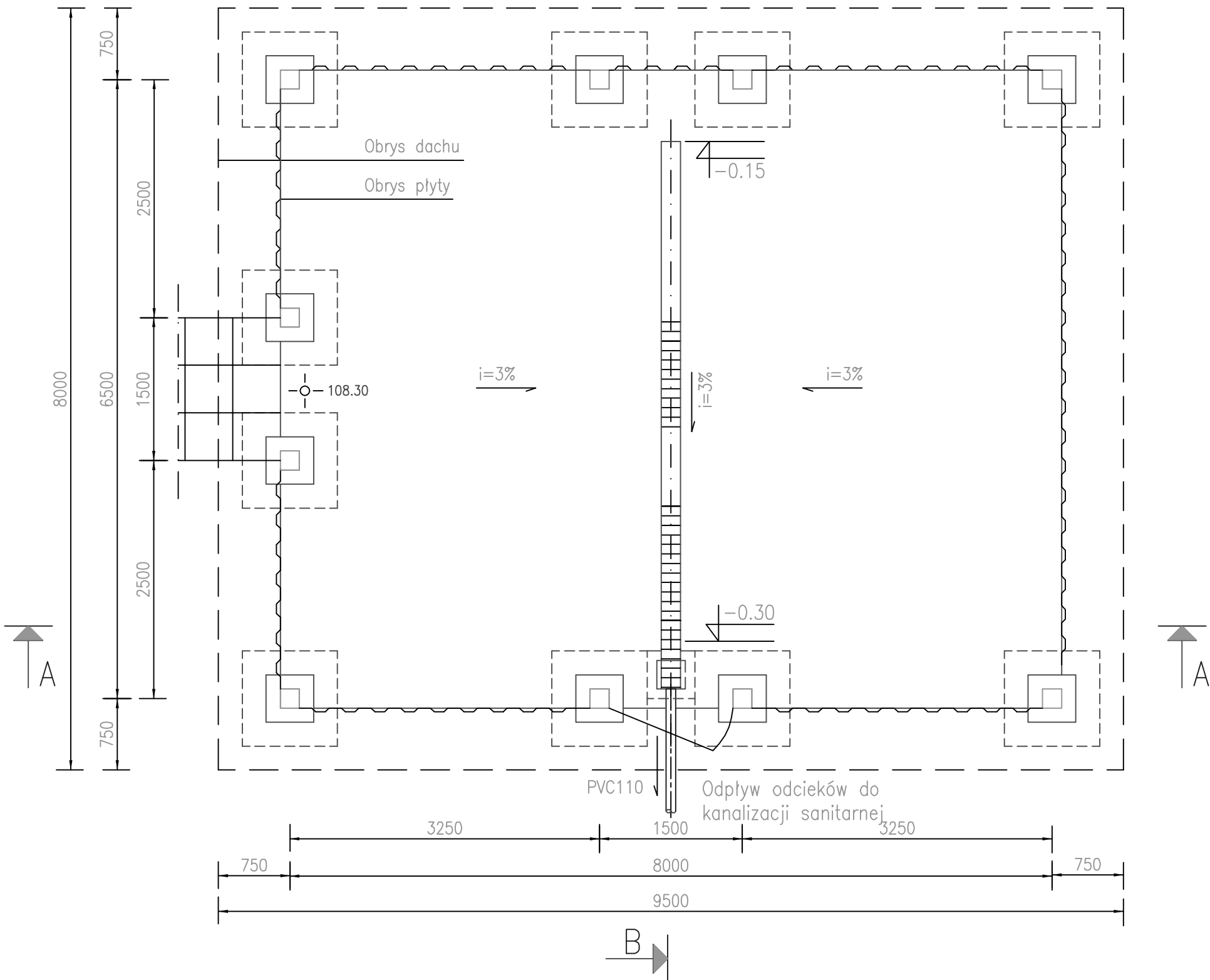
B RZUT.
