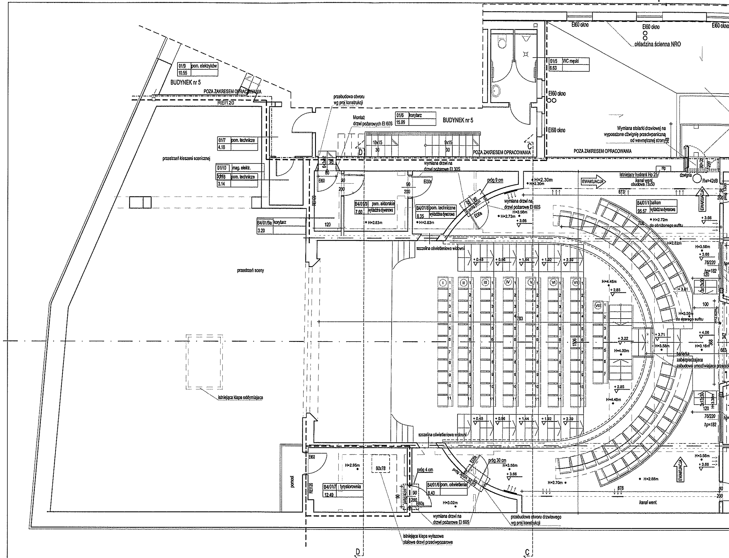
RZUT PIĘTRA: BUDYNEK 4
