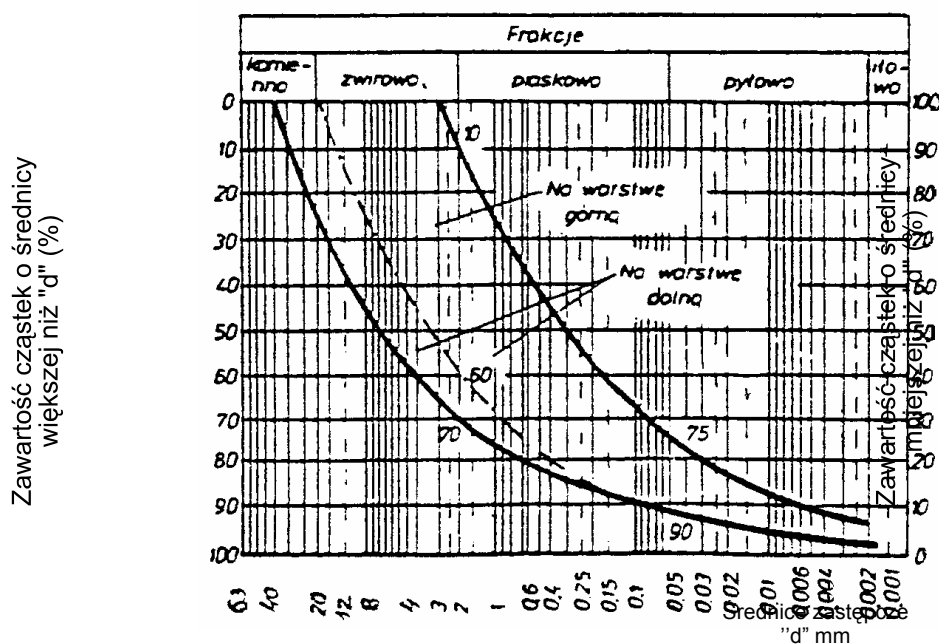
Rysunek 2. Obszar uziarnienia optymalnych mieszanek gliniasto-żwirowych
