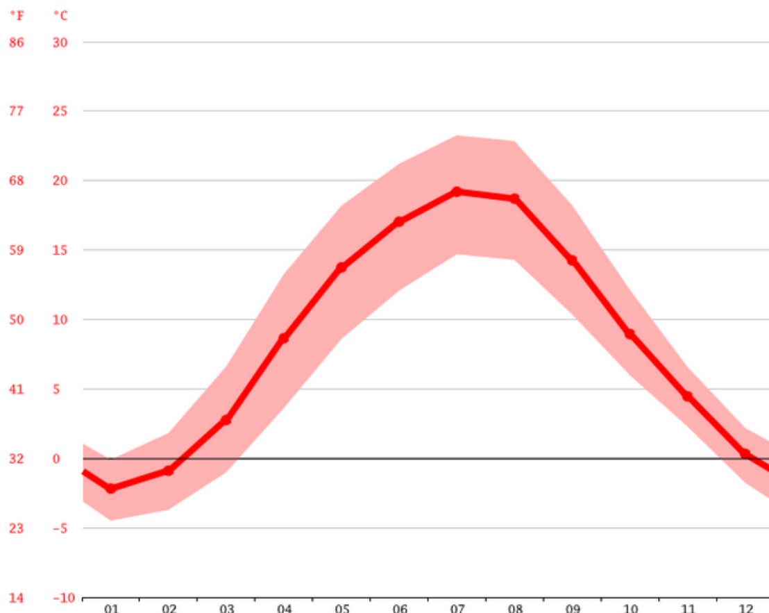
Rysunek 27. Wykres temperaturowy dla gminy Szczutowo Źródło: opracowanie własne na podstawie www.climate-data.org
