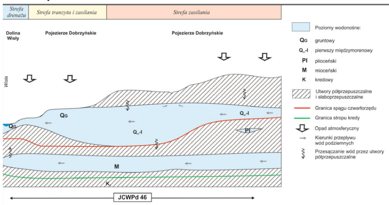
Rysunek 17. Schemat przepływu wód podziemnych w JCWPd nr 46
