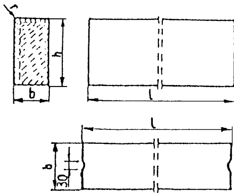
Rys. 1. Wymiarowanie krawężników
