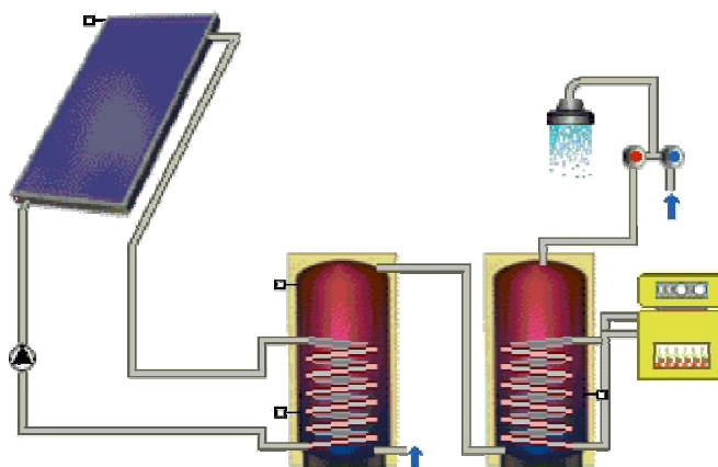
Rysunek 14 Schemat technologiczny przykładowego rozwiązania instalacji solarnej
