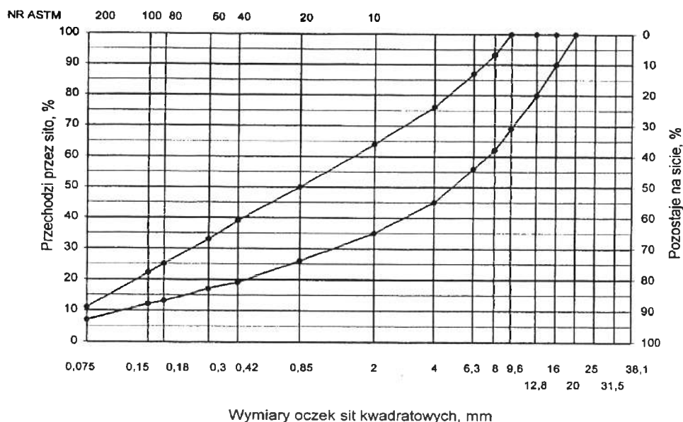
Rys. 1. Krzywe graniczne uziarnienia mieszanki mineralnej BA od 0 do 16mm, od 0 do 12,8 mm do warstwy ścieralnej nawierzchni drogi o obciążeniu ruchem KRI lub KR2
