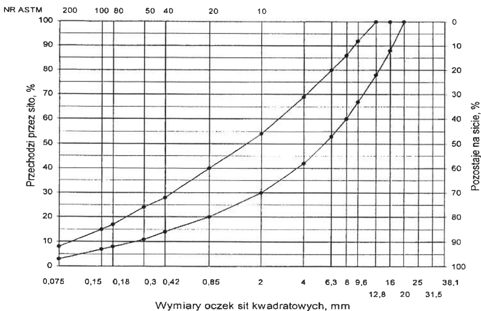
Rys. 2. Krzywe graniczne uziarnienia mieszanki mineralnej z BA od 0 do 16 mm do warstwy wiążącej drogi o obciążeniu ruchem KR1 lub KR2
