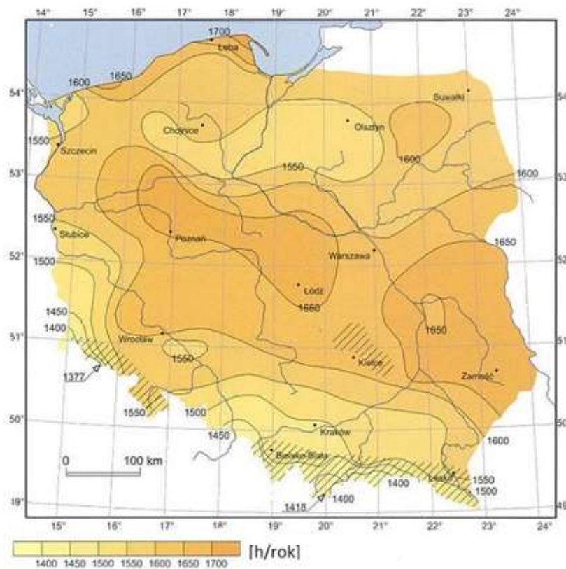
Rysunek 38. Średni czas następcznienia w ciągu roku na terenie Polski [h/rok] [46].
