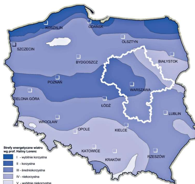
Rysunek 37. Strefy energetyczne warunków wiatrowych [46].
