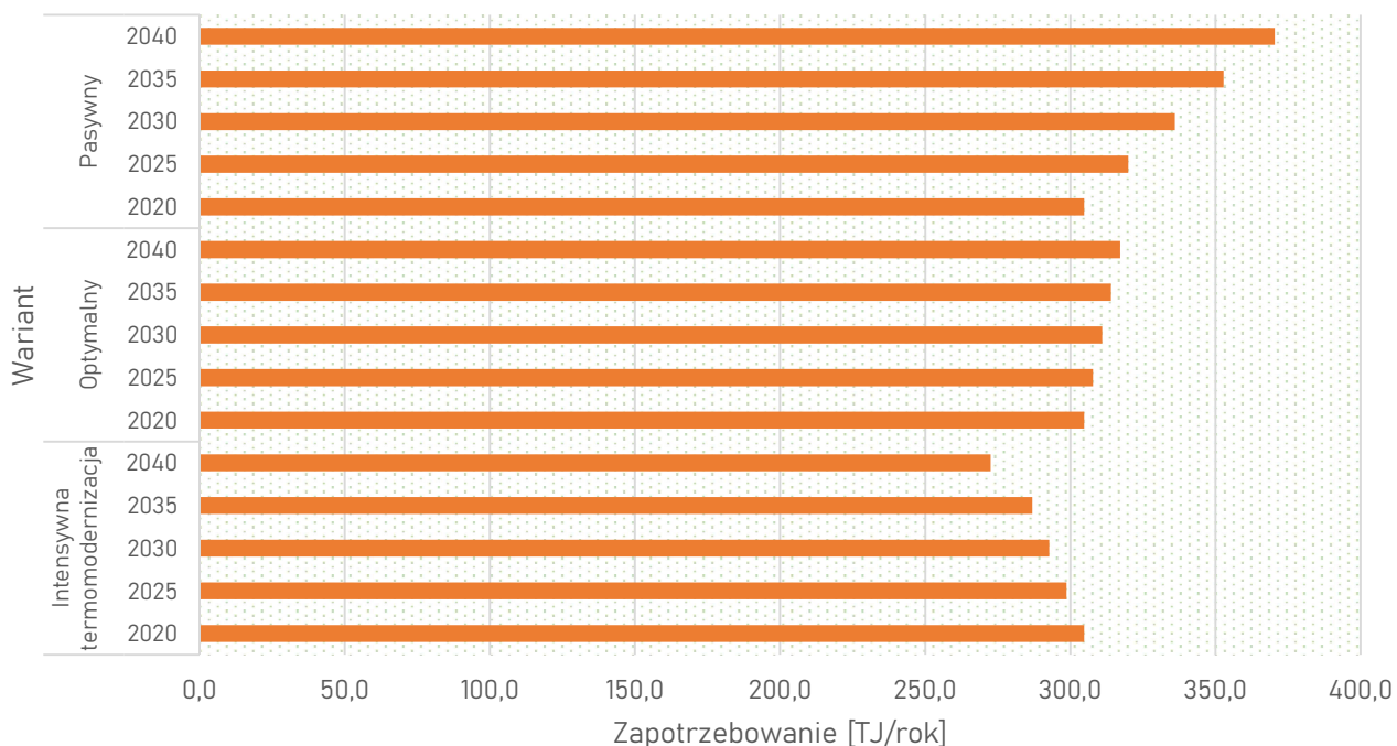
Rysunek 47. Wariantowa prognoza zapotrzebowania na ciepło w Gminie Sośnicowice.
