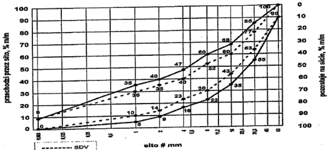
Rys. 2 . Mieszanka niezwiązana 0/63mm do warstwy podbudowy zasadniczej
