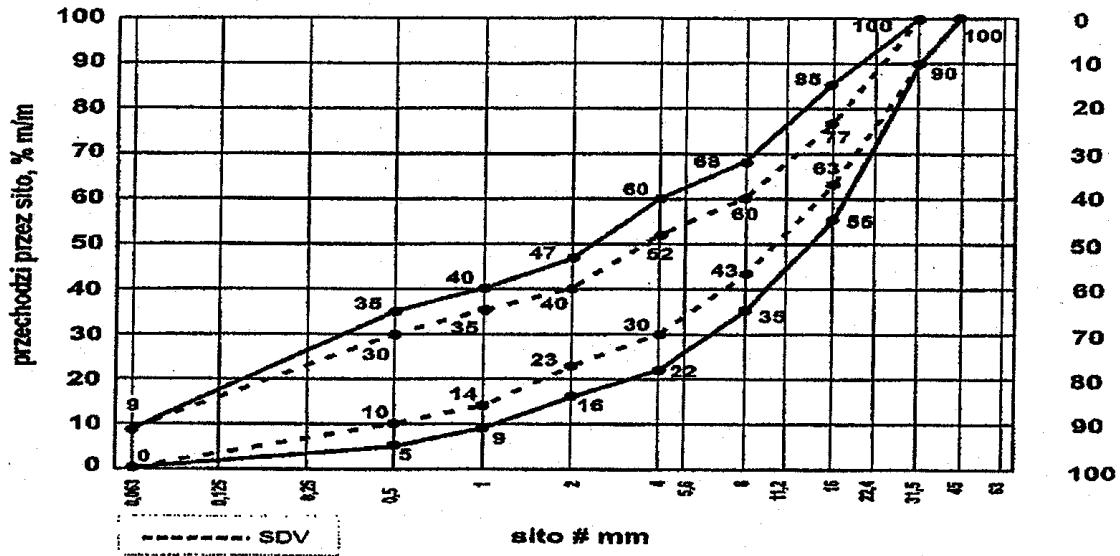
Rys. 1 . Mieszanka niezwiązana 0/31,5mm do warstwy podbudowy zasadniczej
