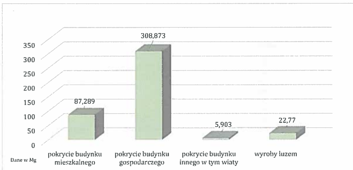
Rysunek 4 Ilość wagowa wyrobów zawierających azbest z podziałem na pokrytą powierzchnię na budynkach mieszkalnych, gospodarczych i innych na terenie gminy Sośnicowice
