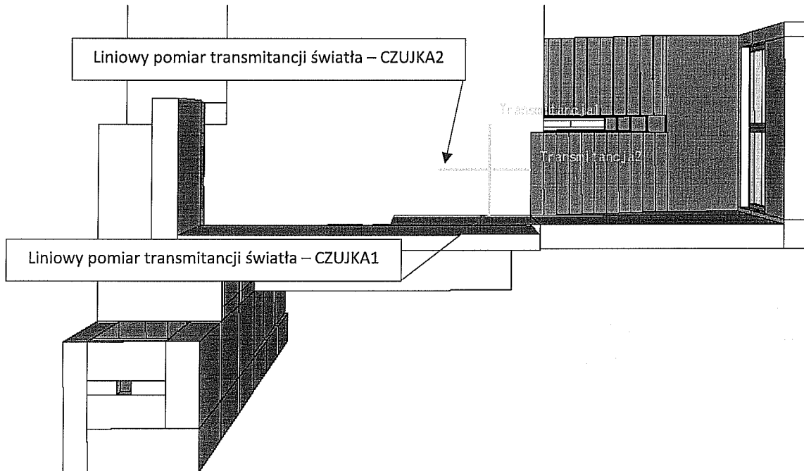
Rys. 8.2. Rzut ostatniej kondygnacji z lokalizacją liniowych pomiarów transmitancji
