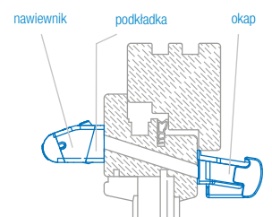
okno drewniane – nawiewnik EMM z okapem akustycznym
