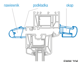
okno PVC – nawiewnik EMM z okapem akustycznym
