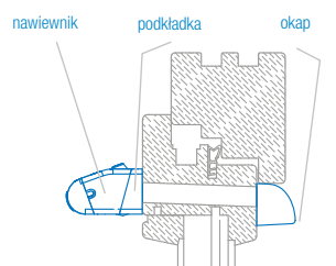
okno drewniane – nawiewnik EMM z okapem standardowym
