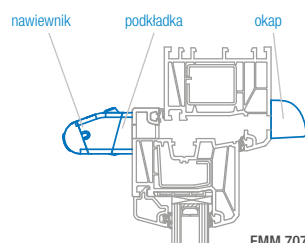
okno PVC – nawiewnik EMM z okapem standardowym
