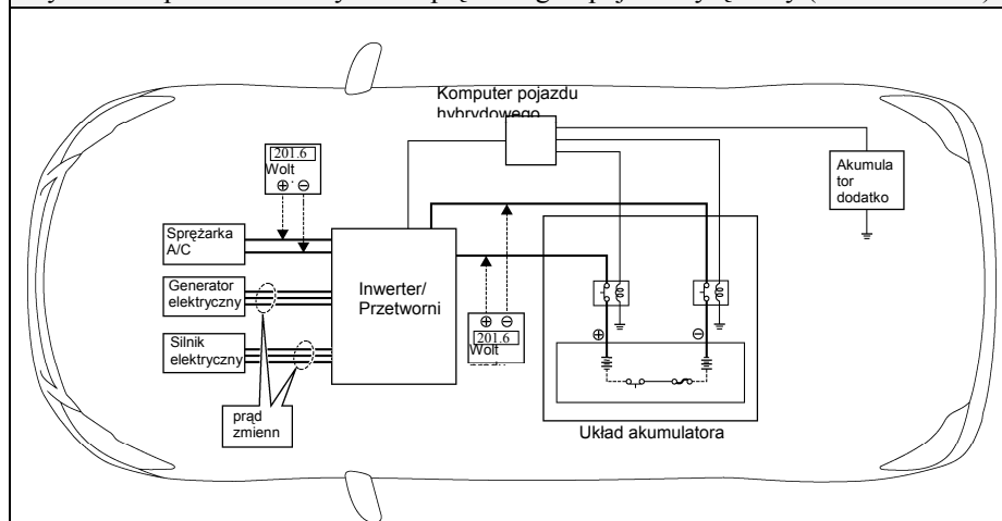
System bezpieczeństwa wysokonapięciowego - pojazd wyłączony (READY-OFF)
