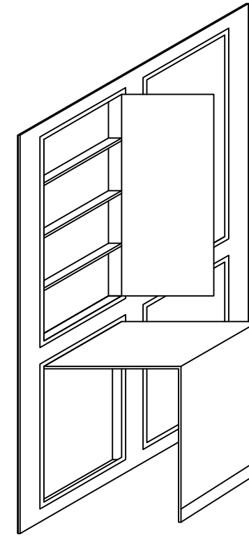
ŚCIANA B - AKSONOMETRIA
