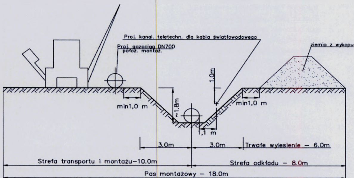
Rys.4. Poglądowy schemat zagospodarowania pasa montażowego - tereny leśne
