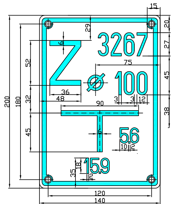
Tablica orientacyjna dla zasuw PN - 86/B-09700-2
