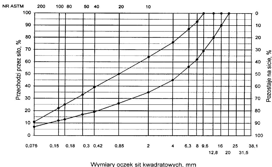
Rys. 1. Krzywe graniczne uziarnienia mieszanki mineralnej BA od 0 do 16mm, od 0 do 12,8 mm do warstwy ścieralnej nawierzchni drogi o obciążeniu ruchem KR1
