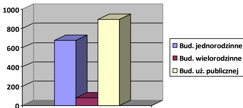
Rys. 20. Redukcja zużycia końcowej energii elektrycznej w poszczególnych typach budownictwa [MWh/rok]
