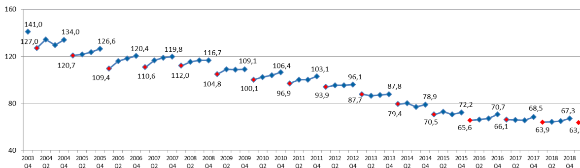
Wykres 3.11 Średnia wartość (w zł) pojedynczej transakcji bezgotówkowej rejestrowanej przez agentów rozliczeniowych w kolejnych kwartałach od IV kwartału 2003 r.
