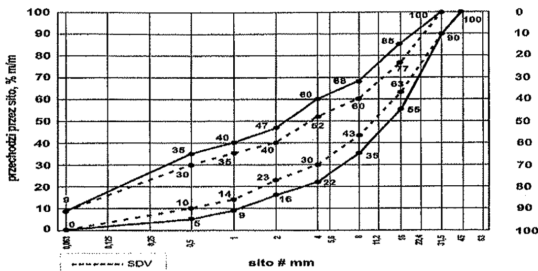
Rys.1 - Mieszanka niezwiązana 0/31,5 mm
