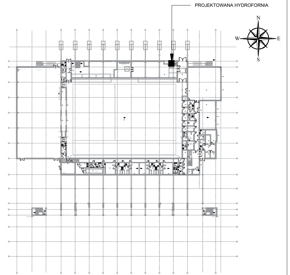
USYTUOWANIE HYDROFORNI - POZIOM -3.60
