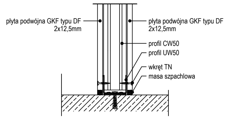
POŁĄCZENIE Z POSADZKĄ
