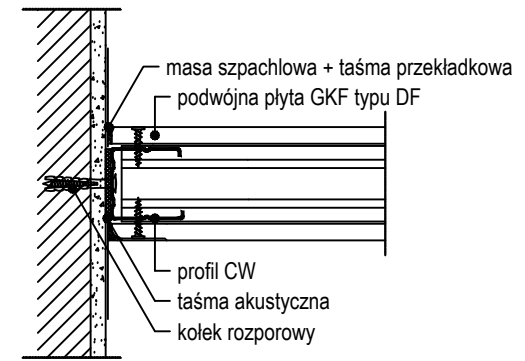
POŁĄCZENIE ZE ŚCIANĄ
